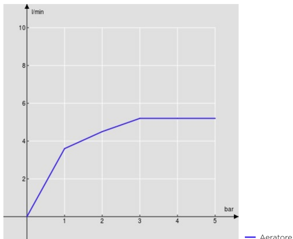
DIAGRAMMA DI PORTATA: ACQUA CALDA/FREDDA
