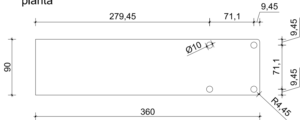
pianta
